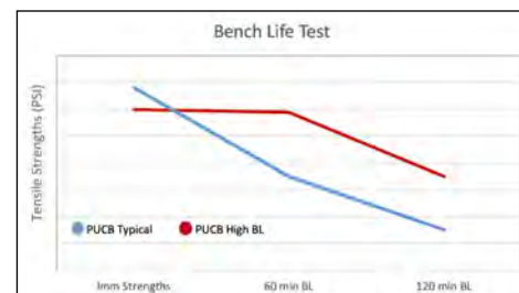
Gráfico 4 - Comparación Bench life a 42CO temperatura de arena & 60% Humedad Relativa. Nivel resina 1,5% relación 55/45 Comp1 a Comp2
